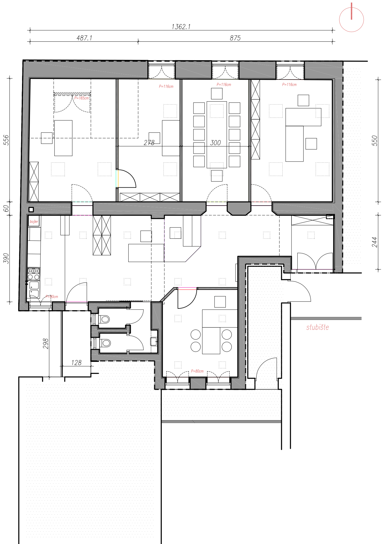
MARTIČEVA 14, IV kat M 1:100
